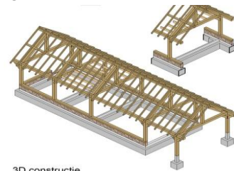
3D constructie
